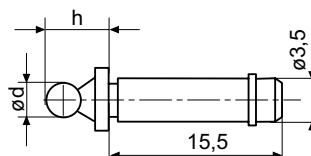
MaraMeter Kugelmess-einsatz
